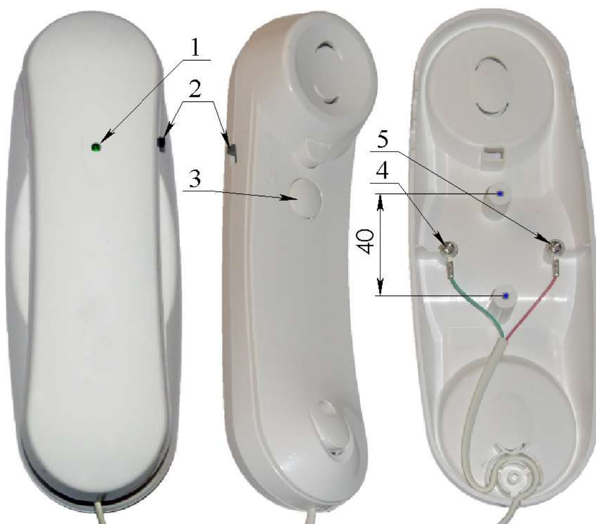
Рис. 1. Расположение органов управления и установочный размер. 1 - индикатор вызова; 2 - выключатель звукового вызова; 3 - кнопка открывания замка; 4 - клемма «-»; 5 - клемма «+».
