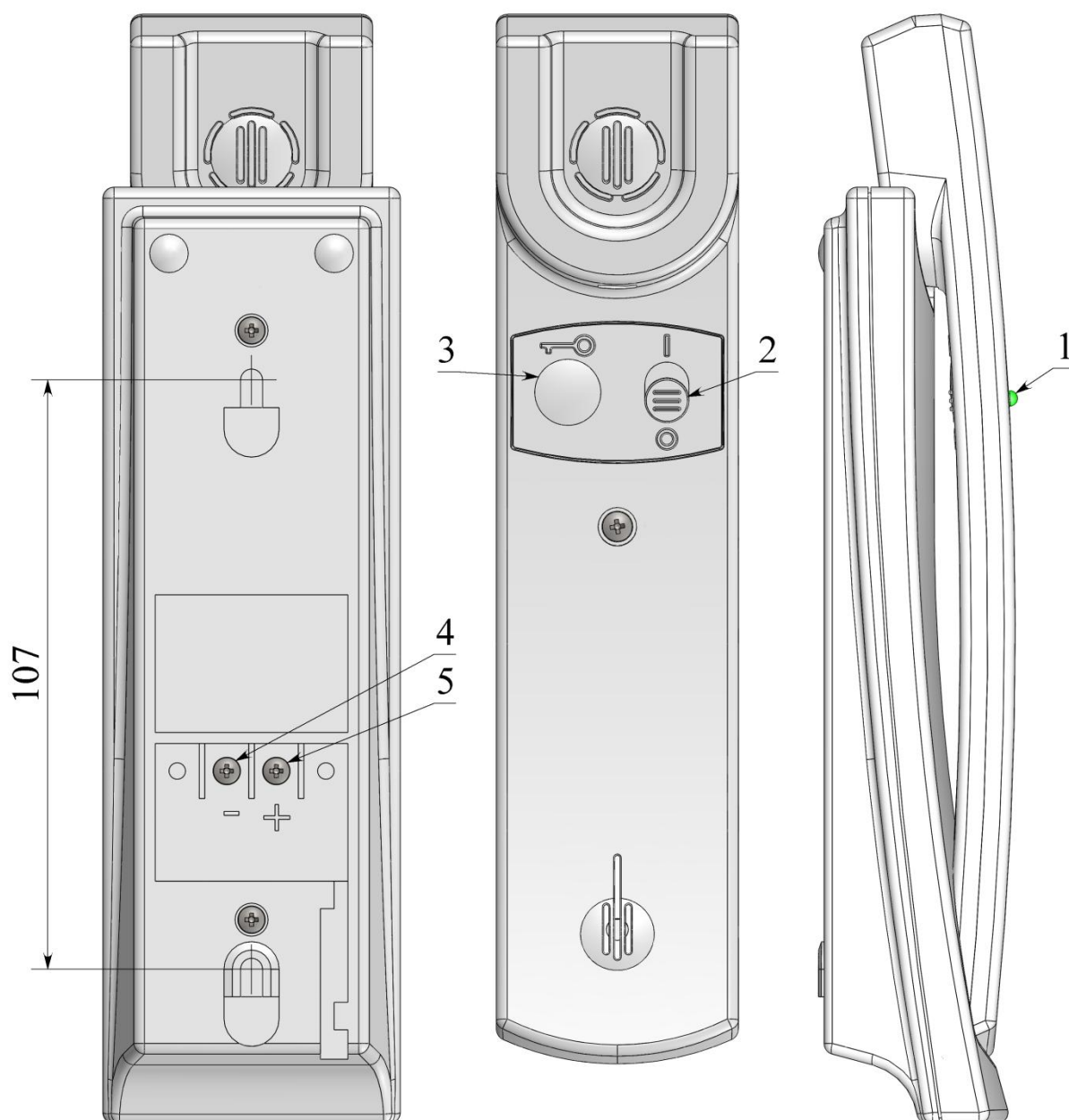
Рис. 1. Расположение органов управления и установочный размер. 1 - индикатор вызова; 2 - выключатель звукового вызова; 3 - кнопка открывания замка; 4 - клемма «-»; 5 - клемма «+».
